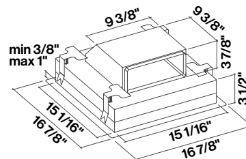
Dimensions de la découpe 15 9/16" x 15 9/16"
